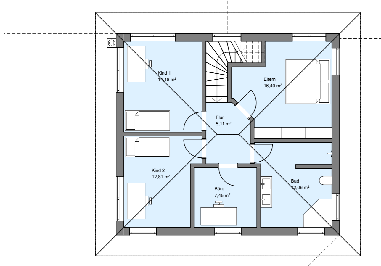
1. Grundriss Dachgeschoss 1:100
