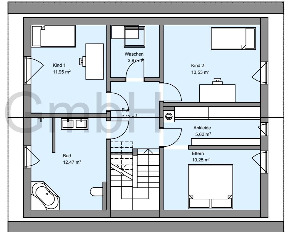
1. Grundriss Dachgeschoss
