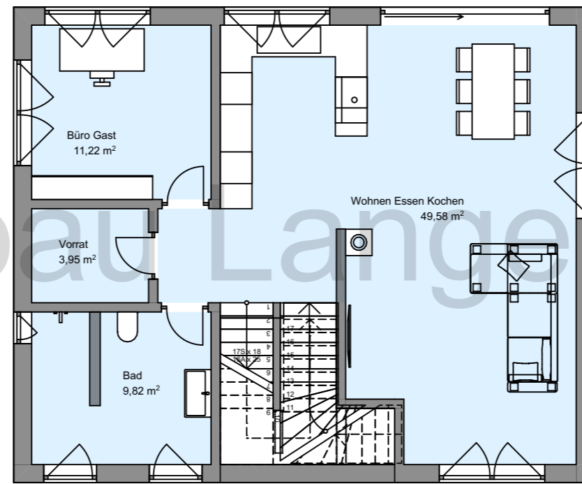
0. Grundriss Erdgeschoss
