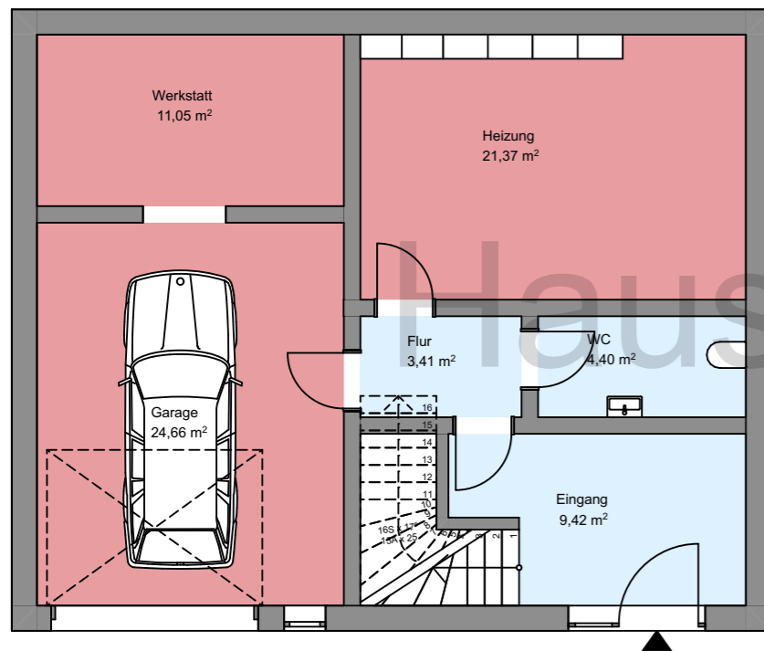
-1. Grundriss Kellergeschoss
